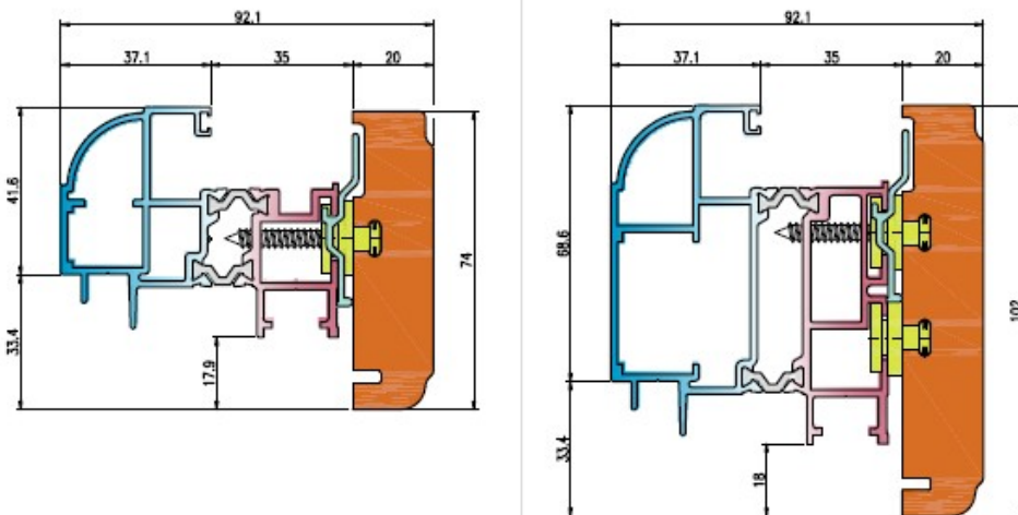
Produzione standard : Sezione ante finestra e porta con vetro ad infilare (non in scala)
