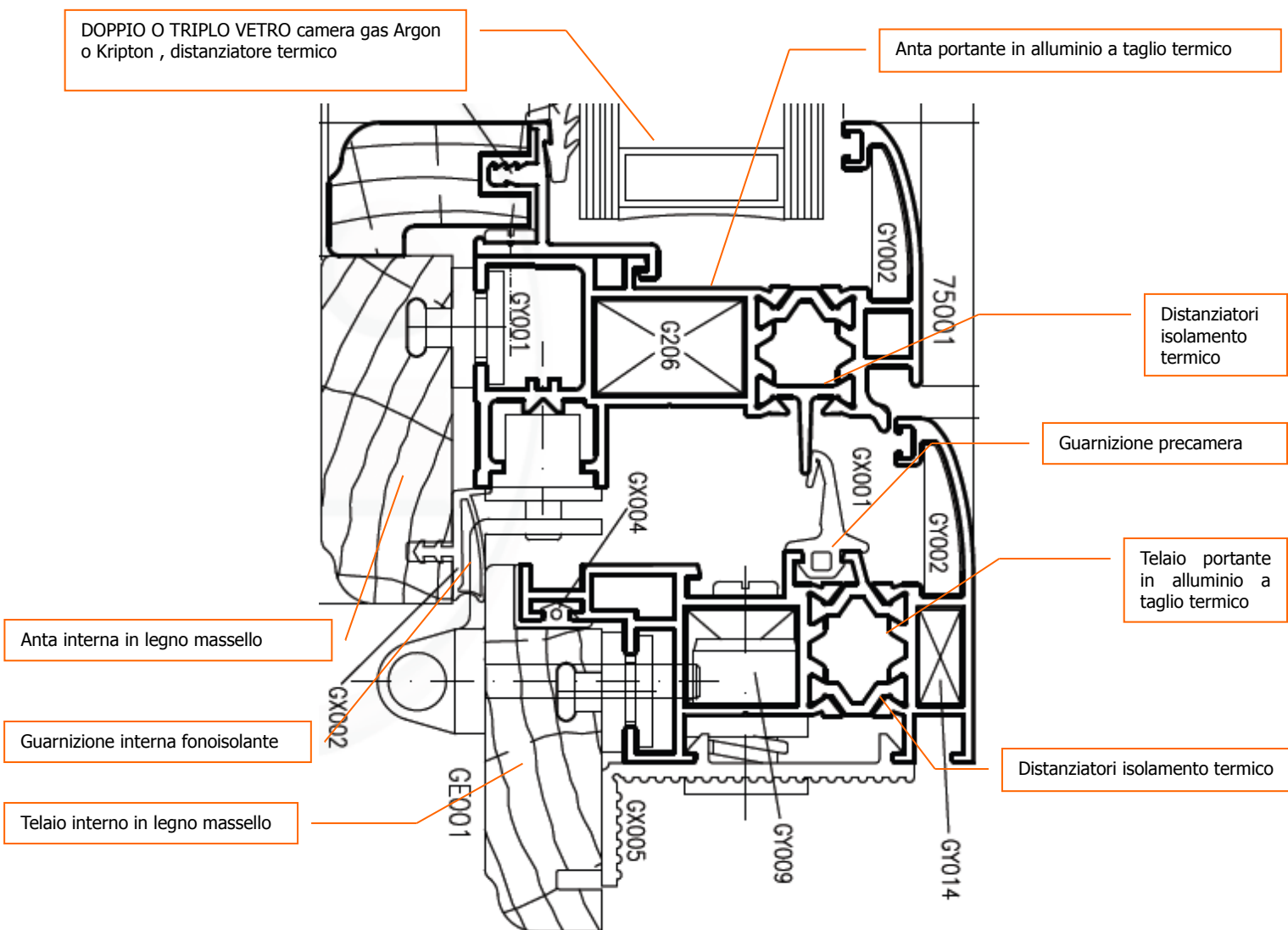
Produzione standard : Sezione ante finestra e porta con vetro ad infilare (non in scala)
